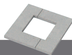
cap i cua | 1200 x 1200 x 80 mm 204 kg
